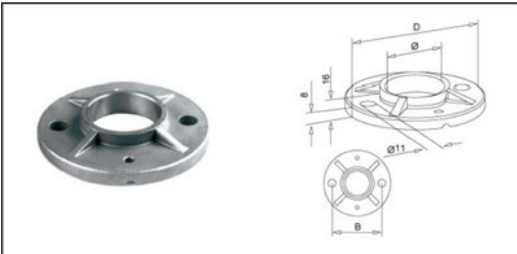
Soporte barra
