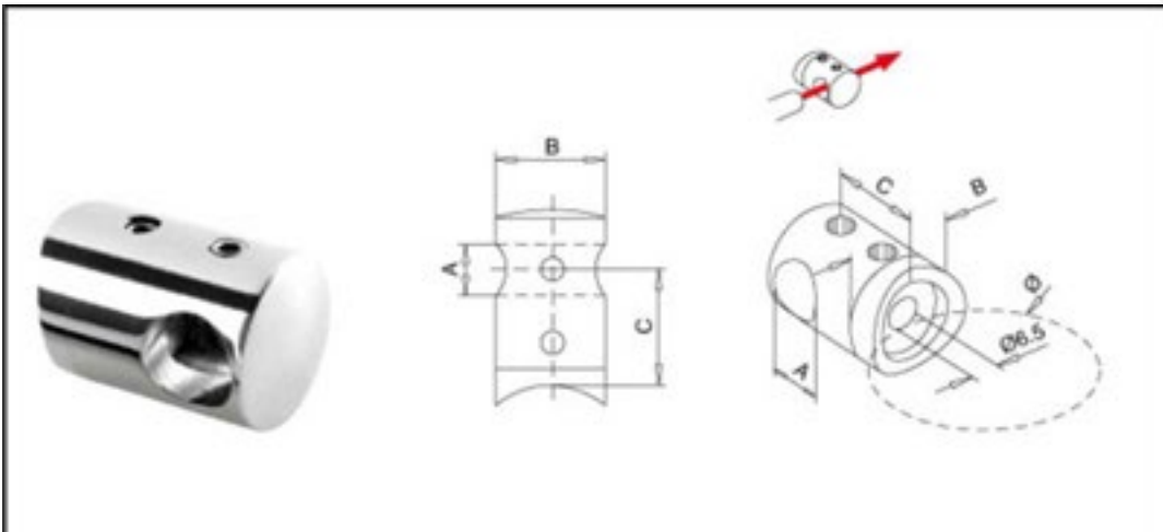
Soporte barra
